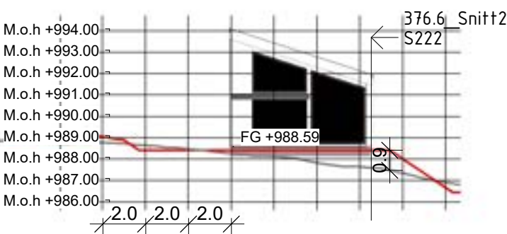
376.6_Snitt1 1 : 250
