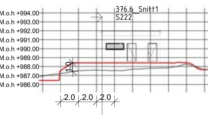
376.6_Snitt2 1 : 250
