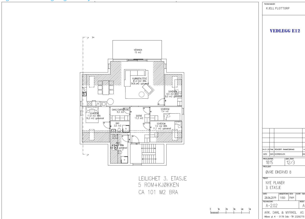
Figur 12 – Plantegning 3. etasje.
